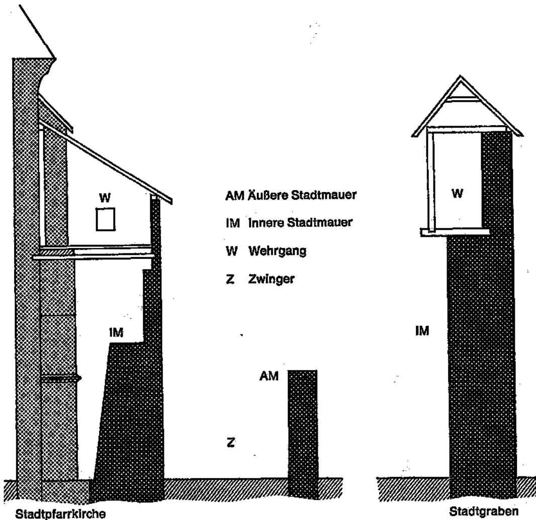
Steyr: Profile der ehemaligen Stadtmauer bei der Pfarrkirche und beim Stadigraben nach Plänen im Stadtarchiv
