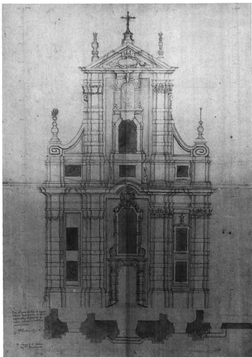
Fassadenaufriss 1690
