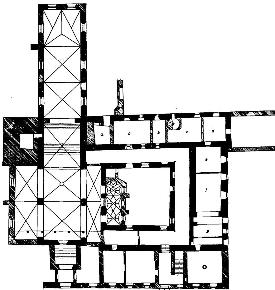
Die Bauanlage des Stiftes Schlägl. gezeichnet von Dr. Anton Macku und Dr. Laurenz Schuster.
