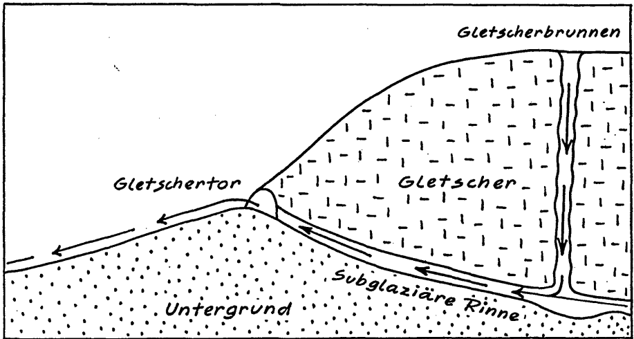
Textabb. 2. Bildung einer subglaziären Rinne
