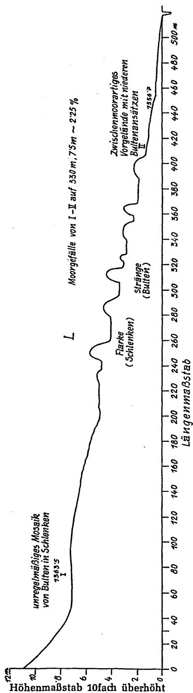
Textabb. 2. Unteres Filzmoos, Längenprofil mit dem Flank-Strang-Komplex. Im Quer = Breitenprofil liegt Süden links.
