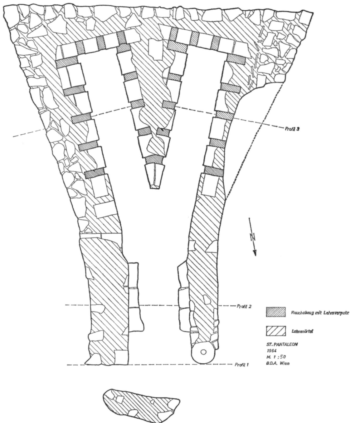
Textabb. 1: Grundriß des Ziegelofens von Erla
