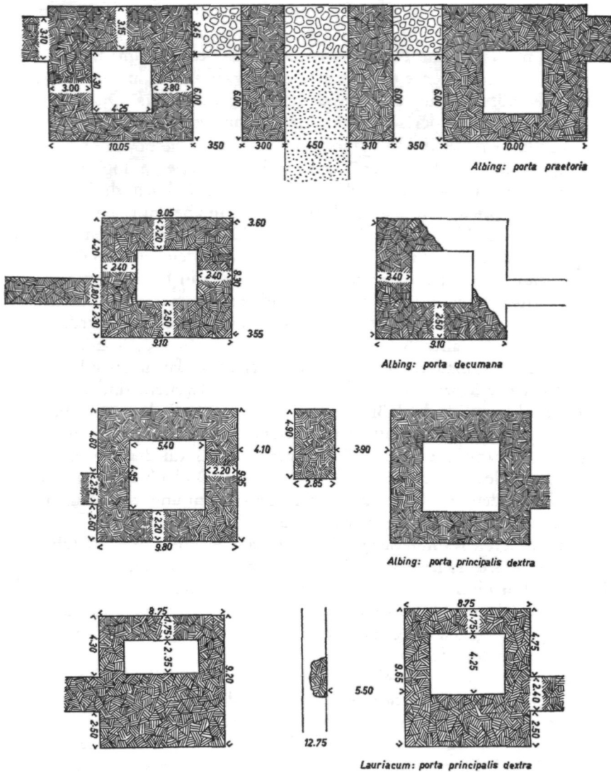
Textabb. 6: Toranlagen der Lager Albing und Lauriacum (Lorch)
