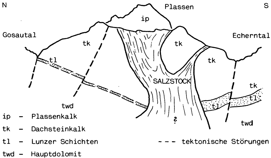
Abb. 5: Der Hallstätter Salzberg als typisch alpinen Salzstock (nach O. SCHAUBERGER)
