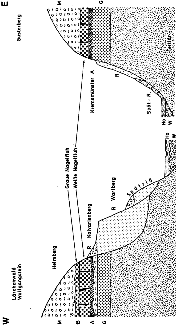
Textabb. 5: Schematischer Querschnitt durch die eiszeitlichen Zungenbecken des oberösterreichischen Kremstales (H. Kohl 1969). Ho = Holozän; W = Würm, periglazial; R = Riß, Moräne u. Schmelzwasserschotter; M = Mindelmoräne, warmzeitl. Bodenbildung A = Kremsmünster A, Bodensediment B = Kremsmünster B; G = Günz, Moräne u. Schmelzwasserschotter.
