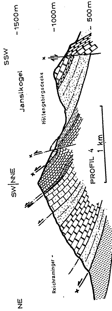
Abb. 6c, d: Geologische Profile durch das Hochsalzgebiet
