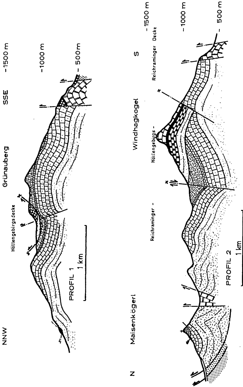
Abb. 6a, b: Geologische Profile durch das Hochsalzgebiet
