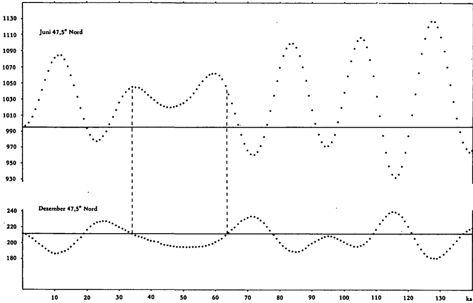
Textabb. 4: Errechnete Insulations-Kurven in unserer geographischen Breite für die Zeit von 140 000 Jahren bis heute. Auf der Ordinate ist die eingestrahelte Sonnenenergie in \text{cal/cm}^2 \text{ d} (Kalorien pro \text{cm}^2 und Tag) eingetragen, die heutigen Werte sind durch horizontale Linien gekennzeichnet (n. DRAXLER & al., im Druck).
