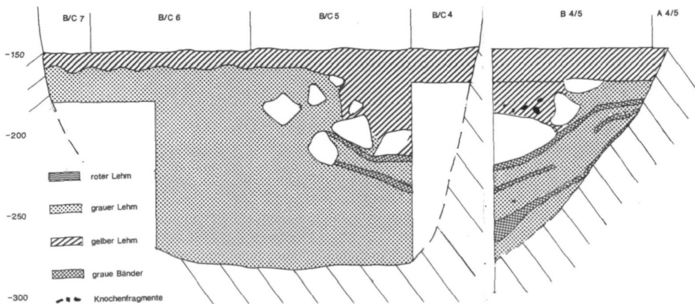
Abb. 3: Quer- und Längsprofil im Kessel.
