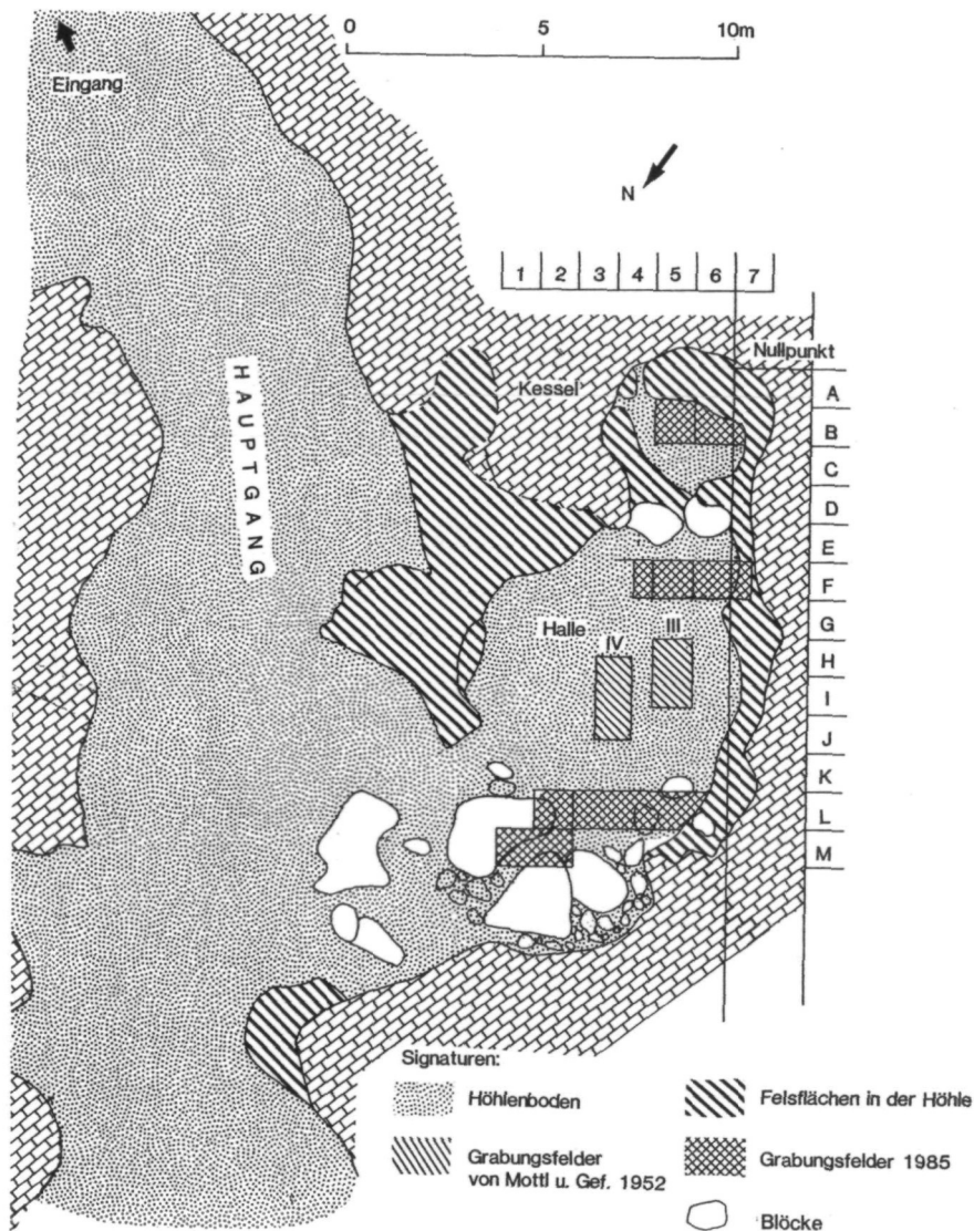
Abb. 1: Grabungsplan der Grabung des OÖ. Landesmuseums im Jahre 1985 in der Bärenhöhle im Kl. Brieglersberg.
