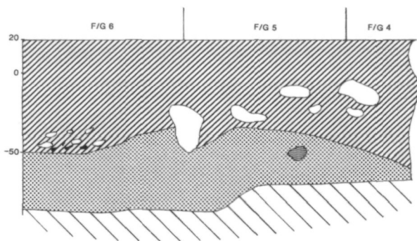
Abb. 2: Querprofil im Bereich der gestörten Sedimente in der Halle. Signaturen s. Abb. 3.
