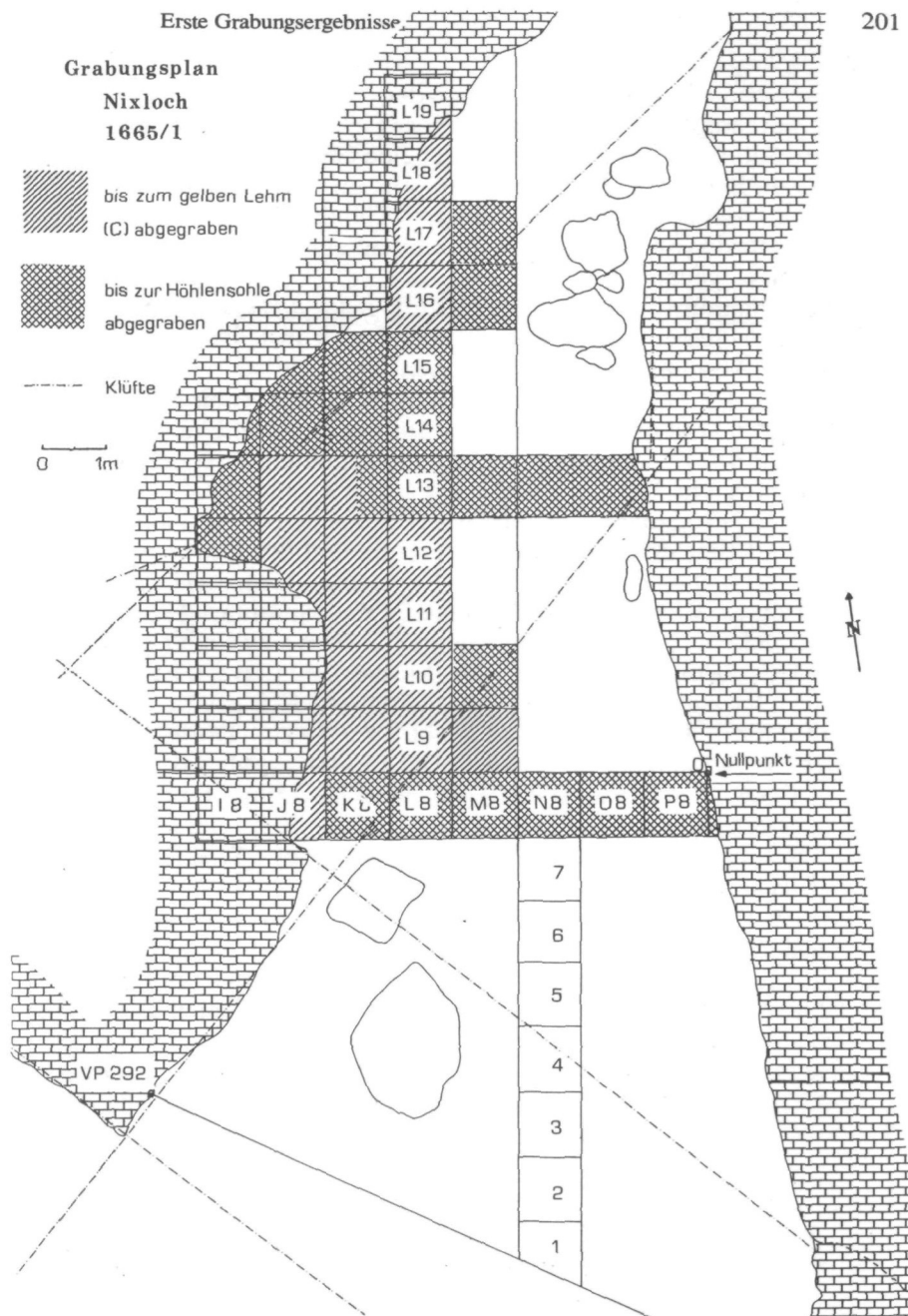
Abb. 2: Grabungsplan des Nixloches — Eingangshalle. Eingetragen sind die gegrabenen Quadranten sowie die tektonischen Klüfte, nach denen die Höhle angelegt ist.
