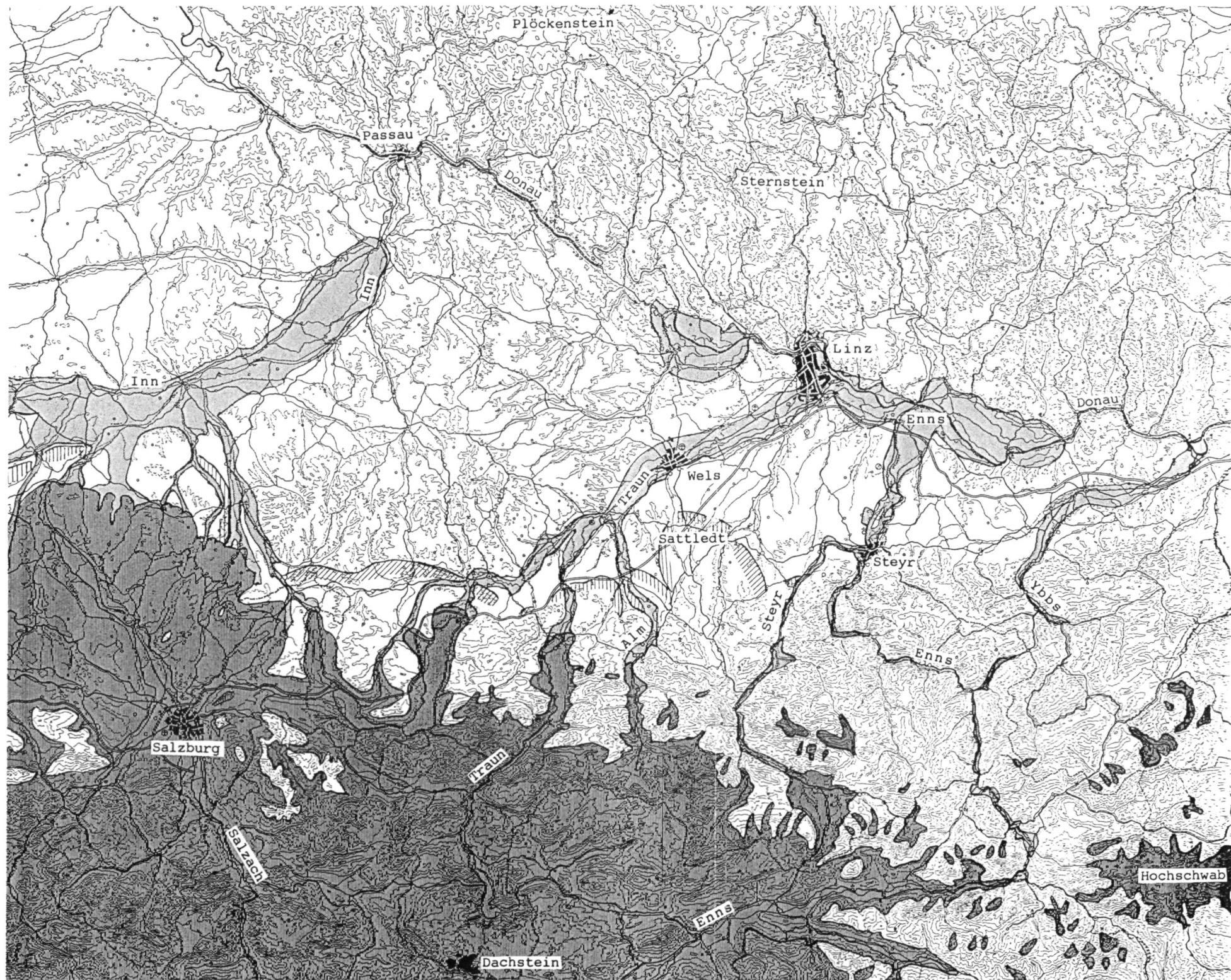
Abb. 3: Die eiszeitliche Verglätscherung der nordöstlichen Alpen
