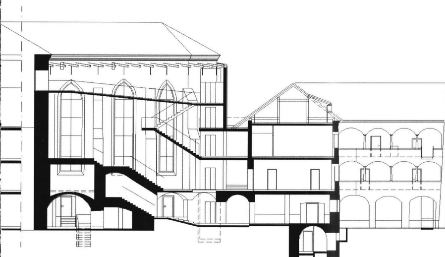
LÄNGSSCHNITTE
