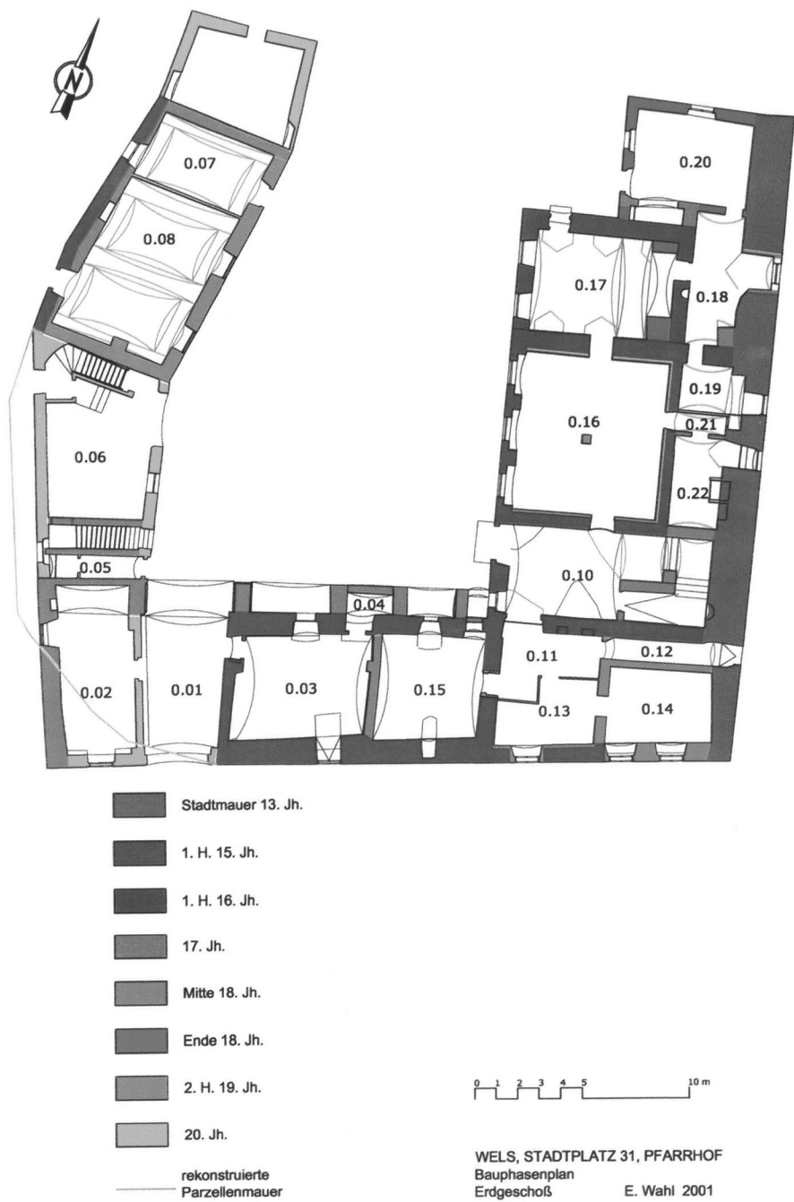
Abb.23 Bauphasenplan Erdgeschoß
