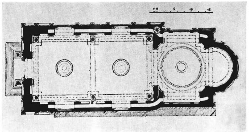
31 Mailand, S. Fedele, Grundriß (Hiersche 1913)
