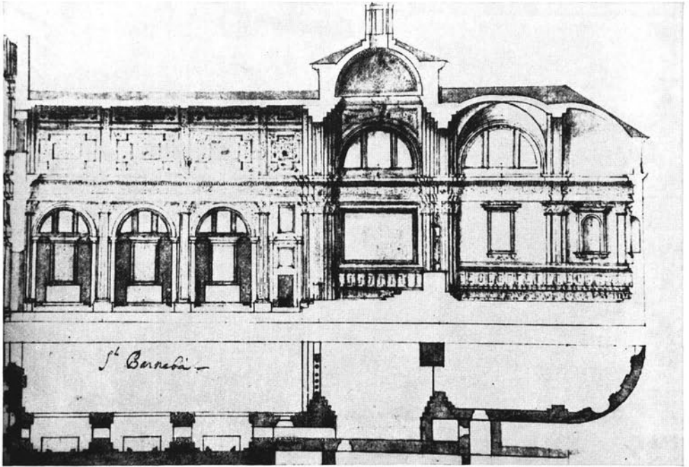
37 Mailand, S. Barnaba, Grundriß und Längsschnitt (Houghton Brown 1964)
