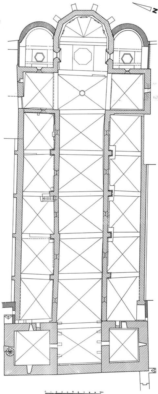
Fig. 3 Dachboden-Grundriß der Stiftskirche von Kremsmünster, Aufnahme Ing. W. Obergottsberger, Ausarbeitung E. Aufreiter, Amt der öö. Landesregierung, Bau6 Vermessung GZAQ36/71, Linz, 17. Dezember 1975
