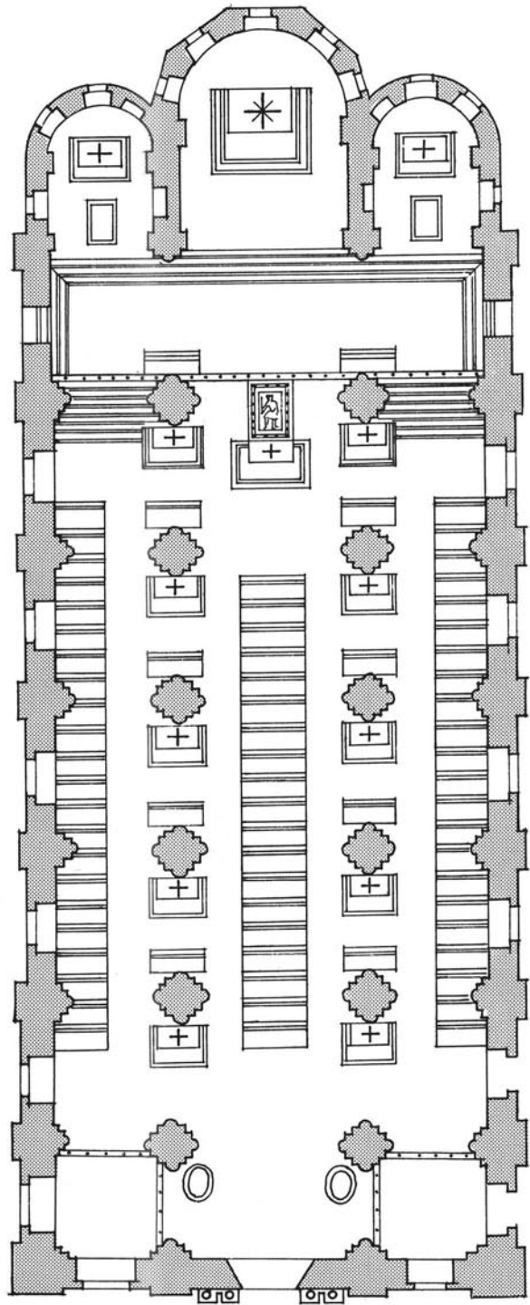
Fig. 1 Grundriß der Stiftskirche von Kremsmünster, Barockisierungs- projekt, 1613/14. Umzeichnung eines auch das Pflaster wiedergebenden Originalplans, Kremsmünster, Stiftsbibliothek
