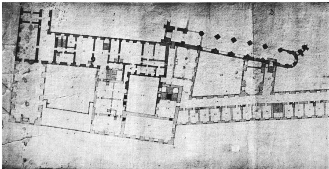
Abb. 2 Stift Kremsmünster, Grundriß des südlichen Teils der Gesamtanlage, erstes Obergeschoß, linker Abschnitt, Projekt von Carlo Antonio Carlone, 1676. Kremsmünster, Stiftsbibliothek
